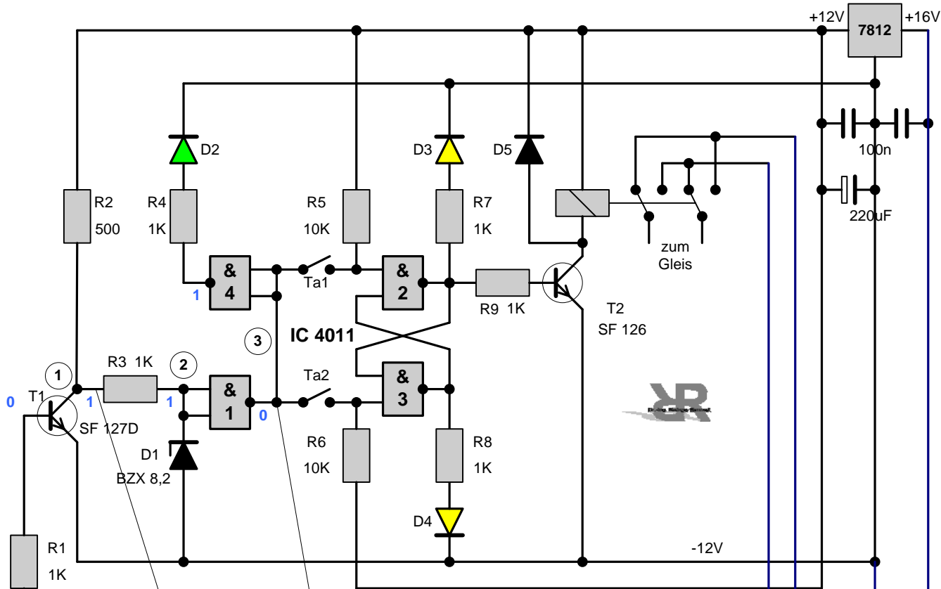
Steuerung Fahrt-Richtungsumschalter
