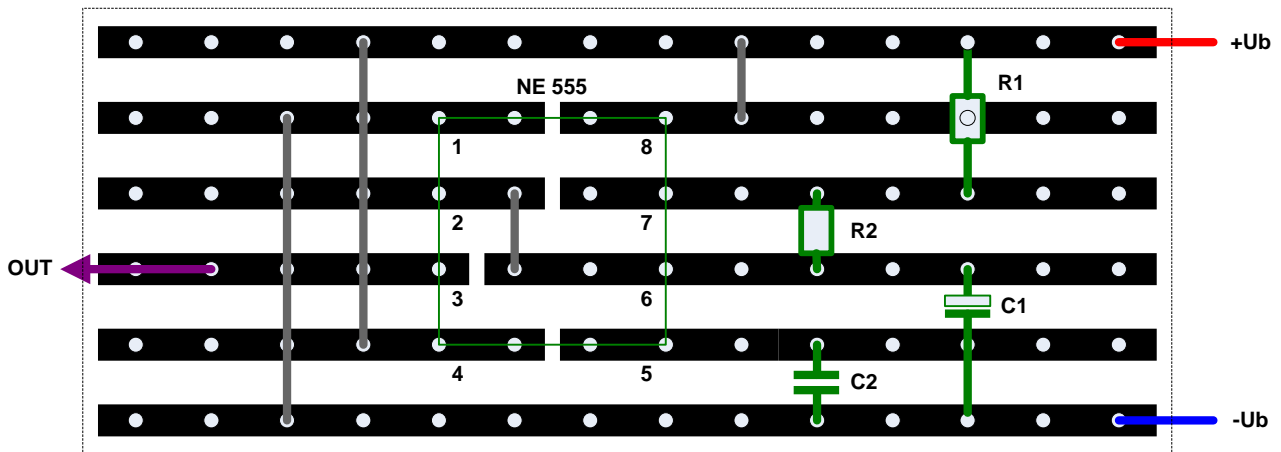
Große Variante ( Bauelementeseite) bel. Kondensatoren und Widerstände
